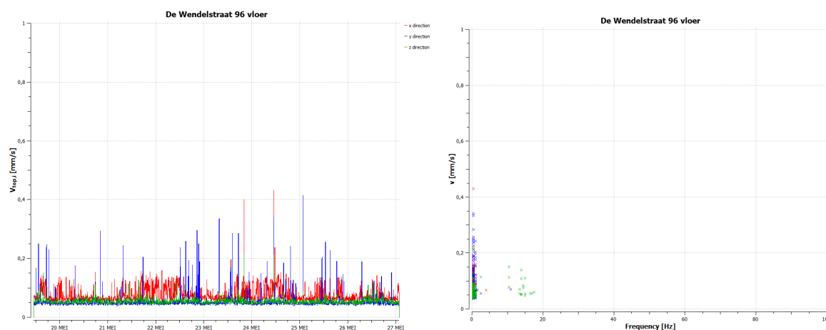
Figuur 4.8: Meetpunt 1, nr 96 vloer, Snelheid versus tijd (links) en versus frequentie (rechts)
