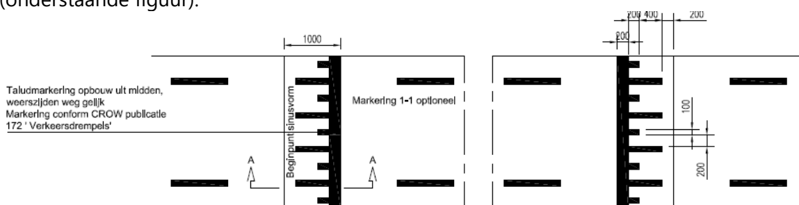
Figuur 5.1: Drempel geometrie (bron CROW)
