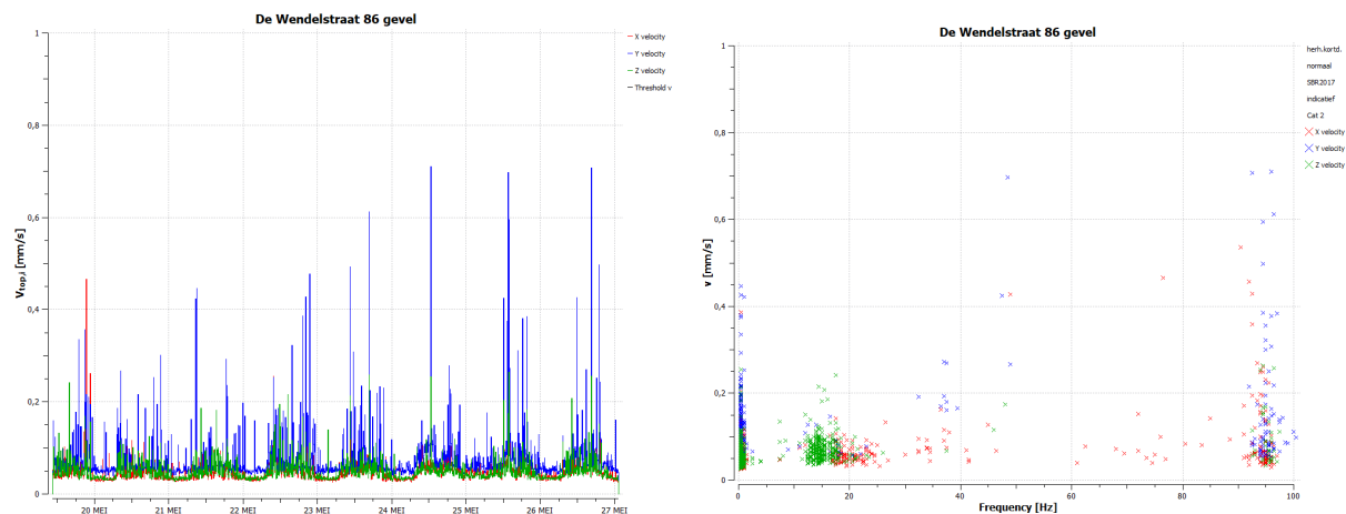
Figuur 4.3: Meetpunt 4, nr 86 gevel, Snelheid versus tijd (links) en versus frequentie (rechts)
