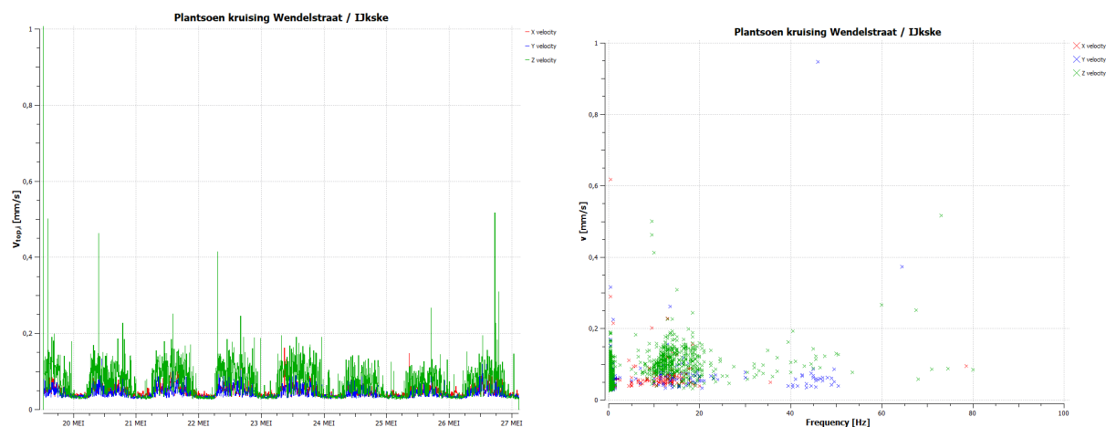
Figuur 4.1: Meetpunt 5, Conus Plantsoen kruising De Wendelstraat / Ijkske Snelheid versus tijd (links) en versus frequentie (rechts)
