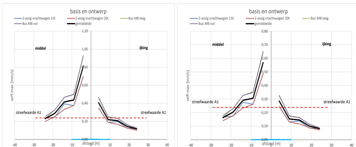
Figuur 5.4: VP-drempel, ijking en klinkers, (links) fundering op staal, (rechts) fundering op palen
