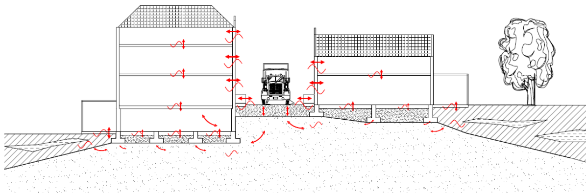
Figuur 2.4: Interacties tussen trillingsbron en ontvanger, situatie fundering op staal
