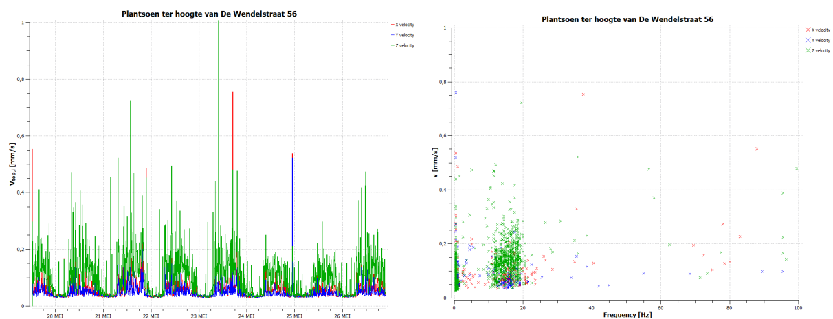
Figuur 4.2: Meetpunt 6, Conus Plantsoen nabij De Wendelstraat 56 Snelheid versus tijd (links) en versus frequentie (rechts)
