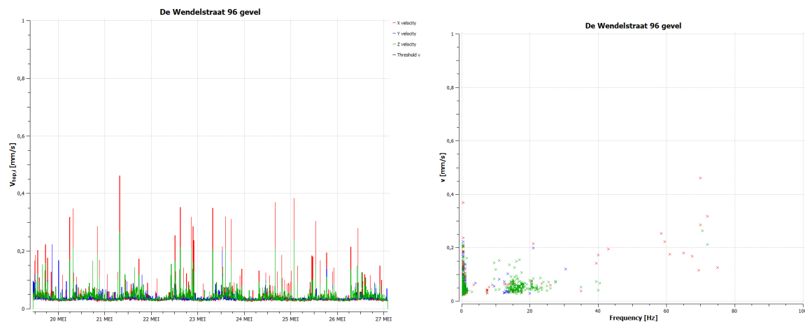
Figuur 4.7: Meetpunt 2, nr 96 gevel, Snelheid versus tijd (links) en versus frequentie (rechts)
