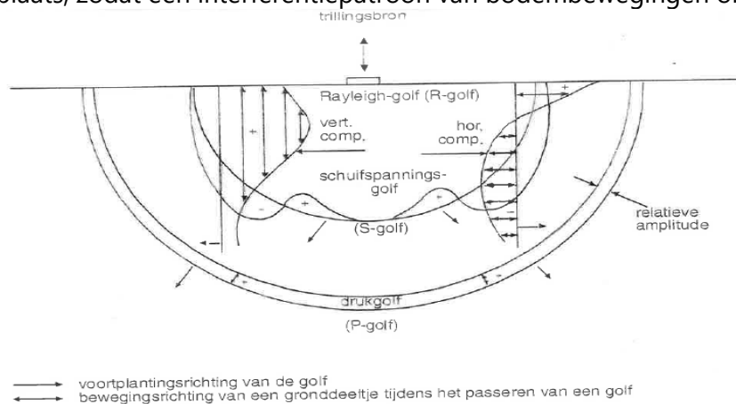
Figuur 2.5a: Verschillende trillingsgolven, verspreiding
