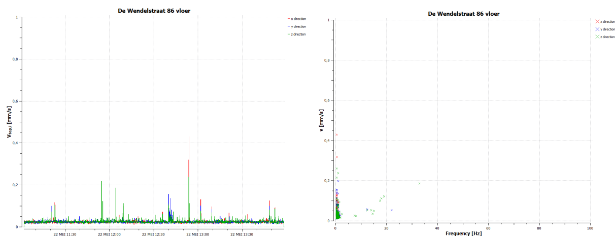
Figuur 4.4: Meetpunt 4, nr 86 vloer, Snelheid versus tijd (links) en versus frequentie (rechts)
