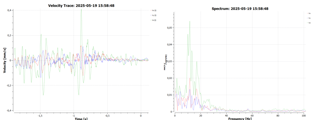
Figuur 4.10: Passage vrachtauto, karakteristieke trillingenbeeld
